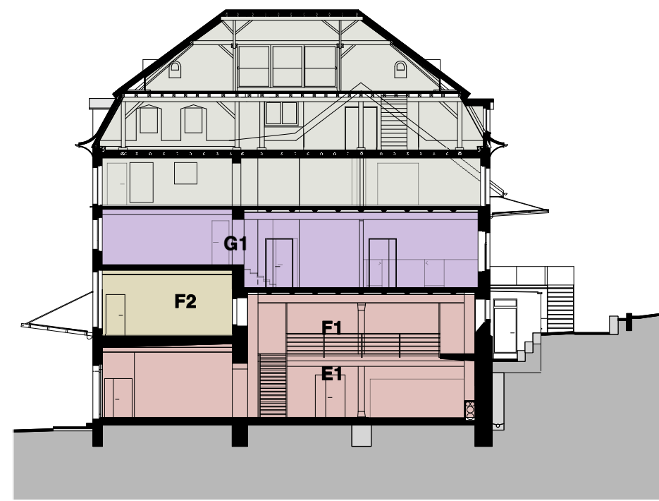
Querschnitt Q3
