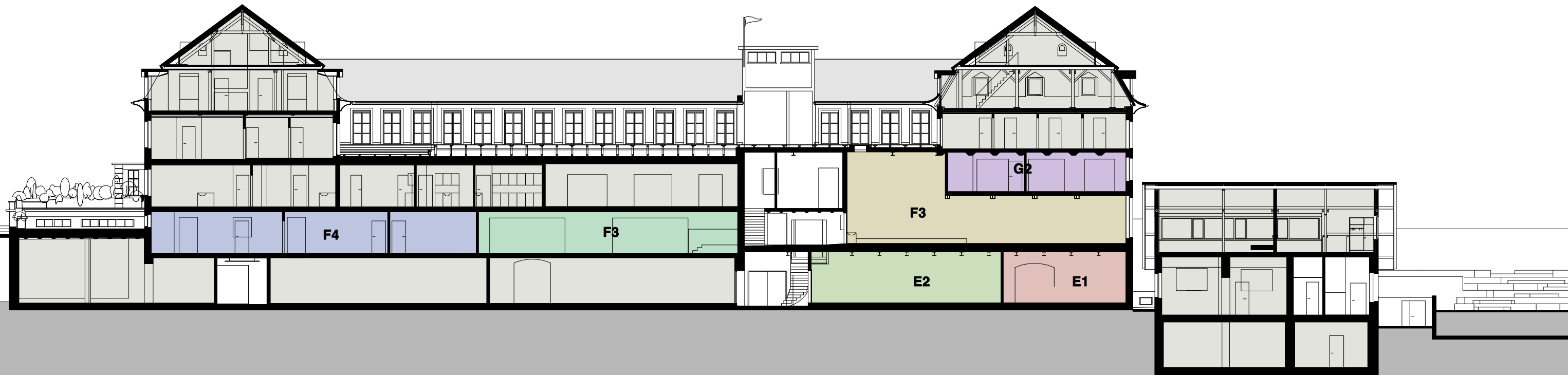
Längsschnitt L1
