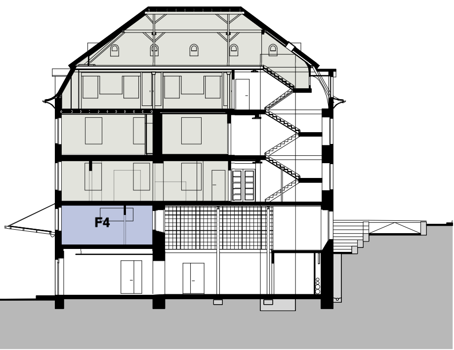
Querschnitt Q1
